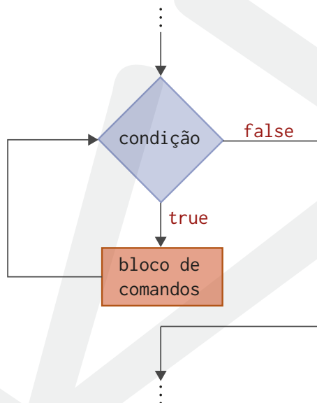
Figura 4.3: Fluxograma da instrução while
