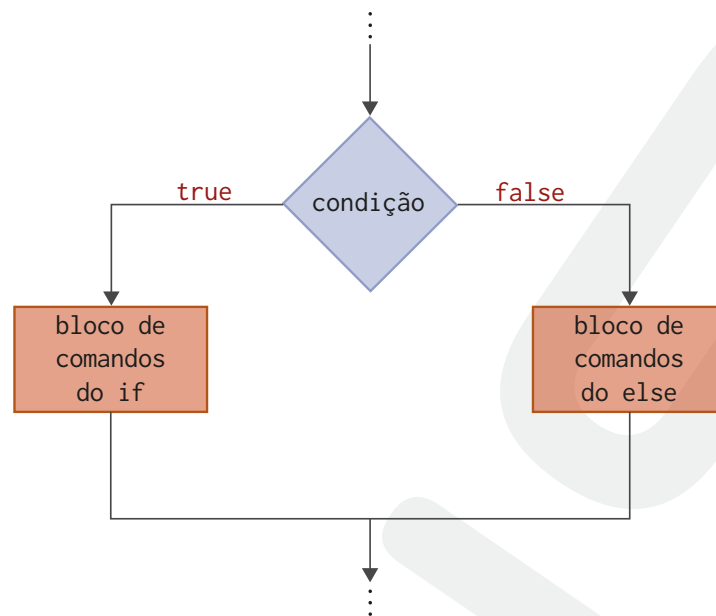
Figura 4.2: Fluxograma das instruções if e else
