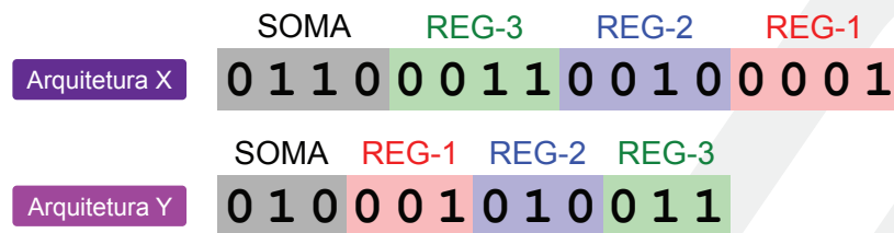
Figura 1.8: Instruções de processadores diferentes
