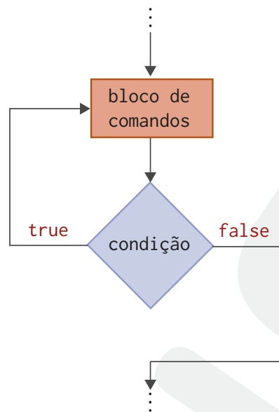
Figura 4.5: Fluxograma da instrução do-while
