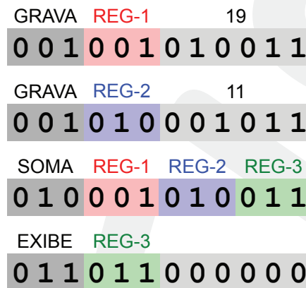
Figura 1.7: Instruções de processador
